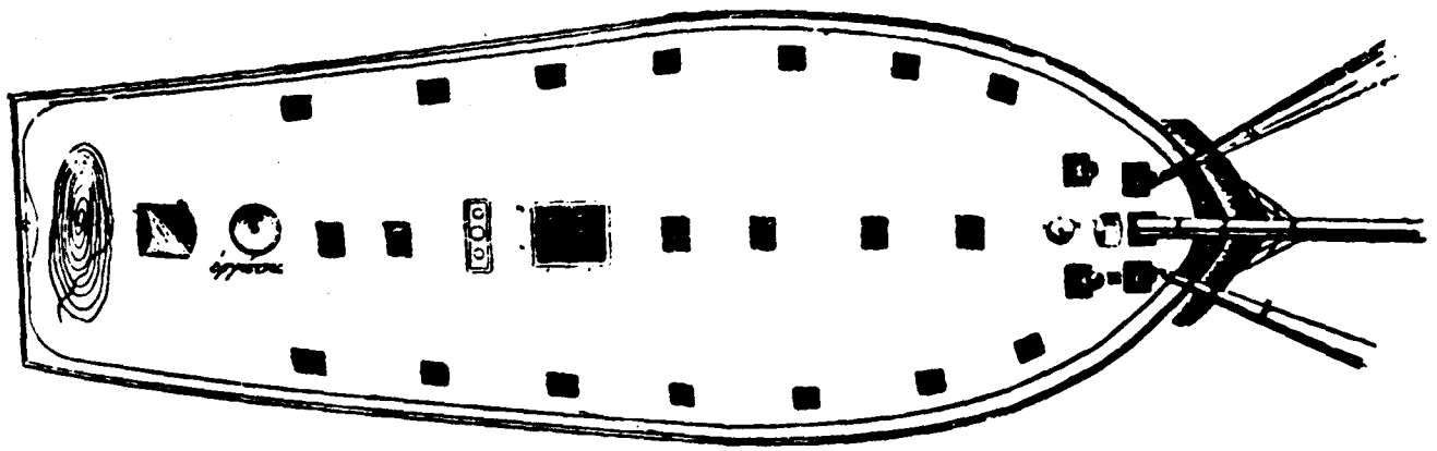
Τύπος ελληνικού πυρπολικού: τὸ κατάστρωμα
